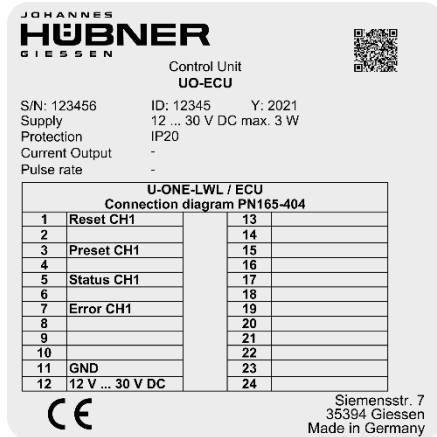
Abb. 4-1: Typenschild (Beispiel)
