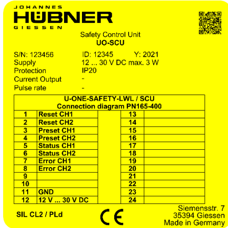
Abb. 4-1: Typenschild (Beispiel)
